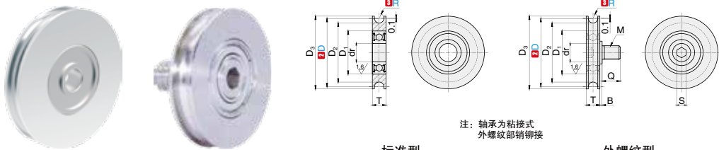
标准型 BRSNN
