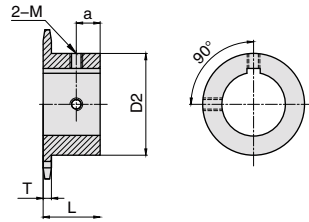
双节距滚子链链轮R型
