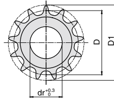
双节距滚子链链轮R型
