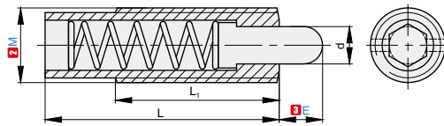
PTSNS 本体无防松 · 钢销型
