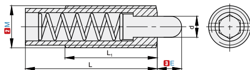
PTSNP 本体无防松 · 塑料销型
