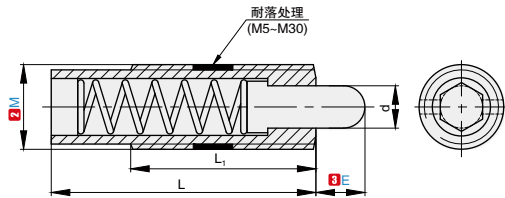
PTSRP 本体有防松 · 塑料销型
