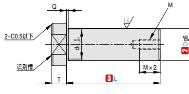
HPEX 内螺纹型
