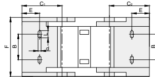
■接头安装尺寸图
