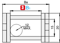
■接头安装尺寸图
