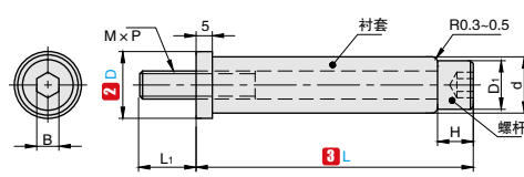
DSPR 直柱型
