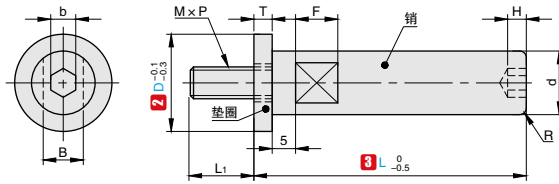
DSP 标准型
