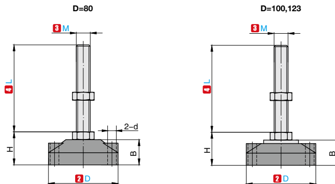
SFNH 安装孔型
